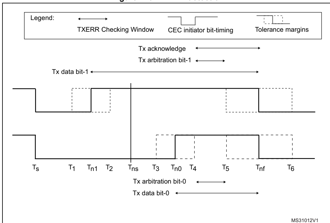
Figure 440. TXERR detection
